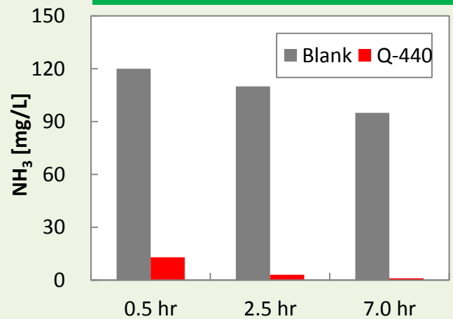
效果(氨性臭味)
