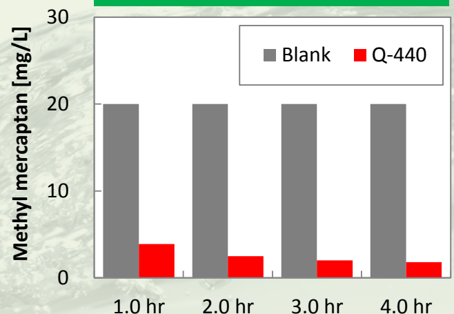
效果(Mercaptan性臭味)
